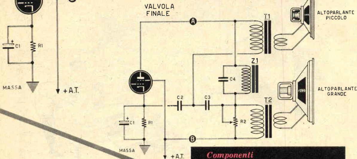
Fig. 2 - Schema elettrico dello stadio amplificatore finale, di un normale ricevitore, modificato con l'aggiunta di un secondo altoparlante di grande diametro atto alla riproduzione delle frequenze basse.
