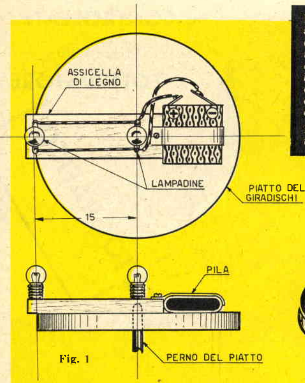
Fig. 1 - Il piatto di un normale giradischi si presta ottimamente per il controllo dei valori bassi della velocità di otturazione della macchina fotografica. Sul piatto giradischi si pone un'assicella di legno sulla quale vengono fissate due lampadine ed una pila. Una delle due lampadine è fissata in corrispondenza del perno del piatto e l'altra è fissata alla precisa distanza di 15 cm. dalla prima.
